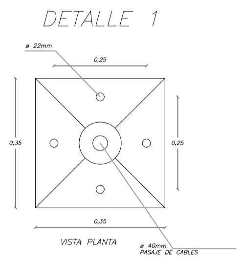
DETALLE ANCLAJE ESCALA 1/10
